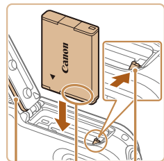
Anschlüsse Dichtungsring Akkuverriegelung
