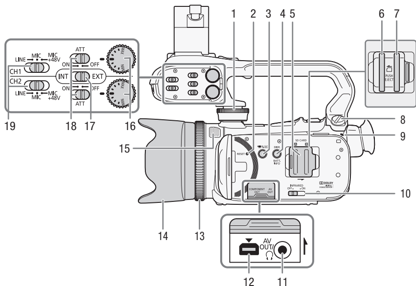
左视图
