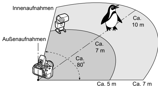
Beispiel für eine drahtlose Blitzanordnung
