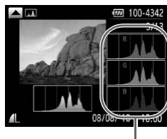
Histogramme RVB
