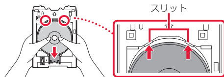
スリット
