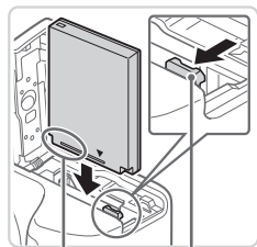
端子部
