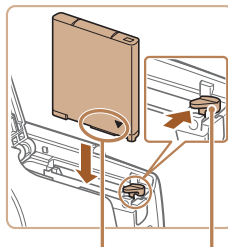
Anschlüsse Akkuverriegelung
