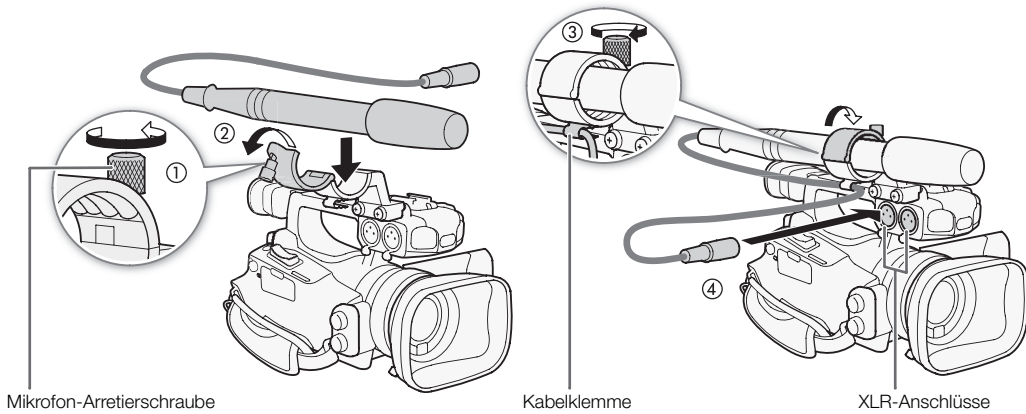
Mikrofon-Arretierschraube
