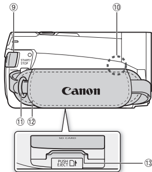
右视图
