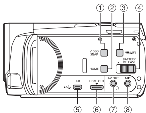
右视图
