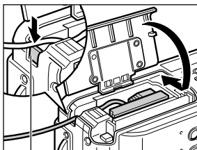
直流电连接器接线盖
