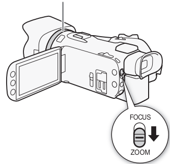
Scharfstell-/Zoomring
