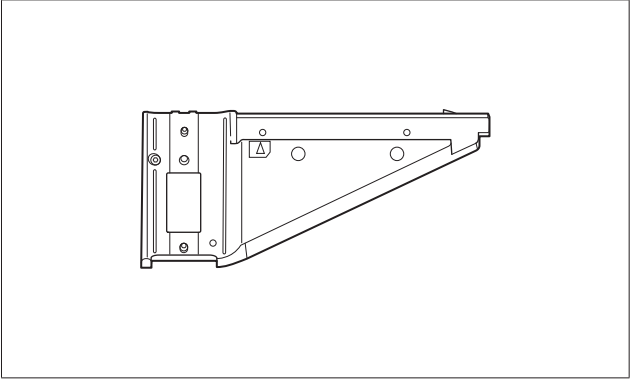
レールユニット L Support rail L Rail de support L Raíl del soporte L Trilho de suporte L Stützscheiene-L Guida del supporto L Steunrail L Podpórka L
