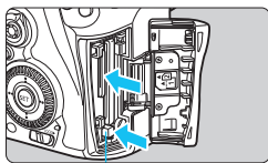
CF-Karten-Auswurfaste
