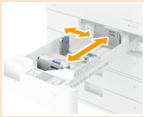
Papierkassette 1 (ISO-C5)
