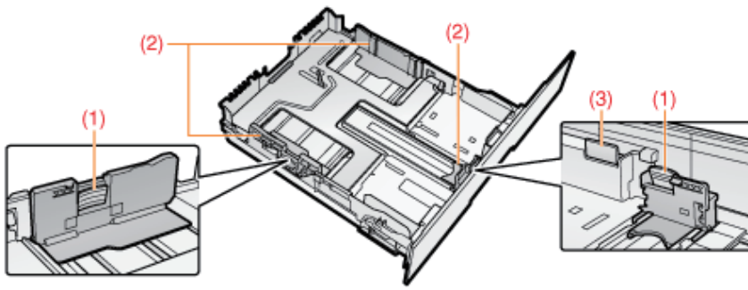
(1) Verriegelungslösehebel (2) Papierführungen (3) Verriegelungslösehebel
