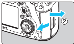
CF卡(卡1)
