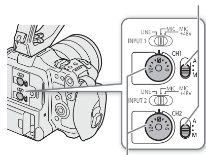
録音レベル調整つまみ
