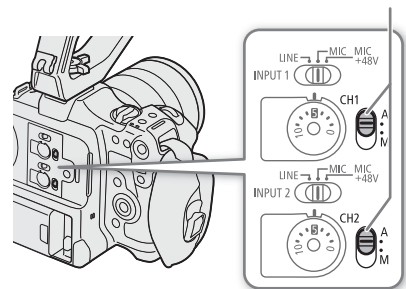
録音レベル切り換えスイッチ
