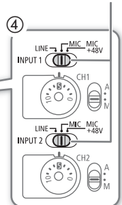
INPUT 1／INPUT 2端子 入力切り換えスイッチ
