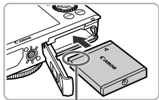
단자
