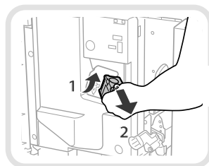
Module de Finition agrafage-J1/ Module de Finition P.A.C.-J1 (En option)
