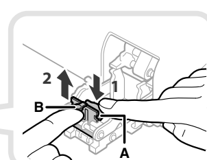
Sattelhefteinheit des Broschüren Finisher J1
