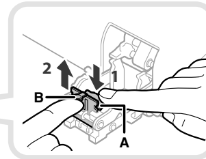
Unità di pinzatura a sella del Booklet Finisher-J1
