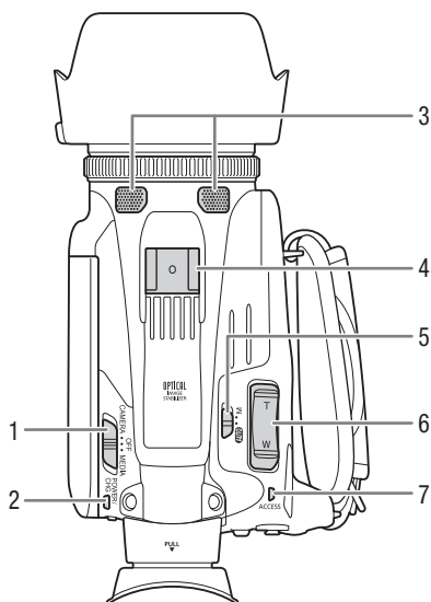
顶视图
