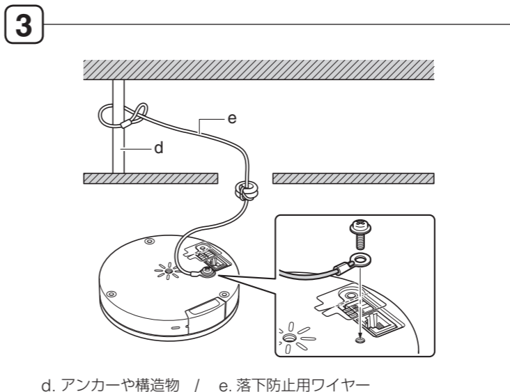
d. アンカーや構造物 / e. 落下防止用ワイヤー
