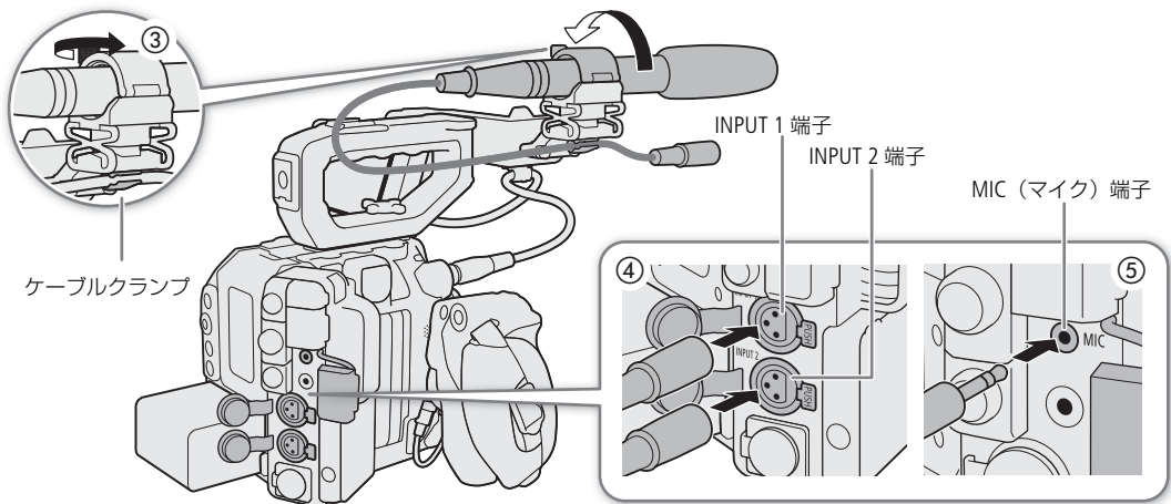
外部マイク固定ネジ
