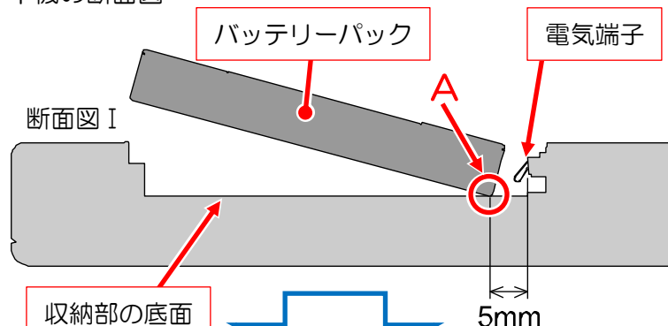
本機の断面図
